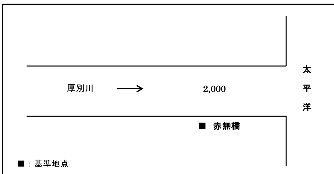
計画高水流量配分図
