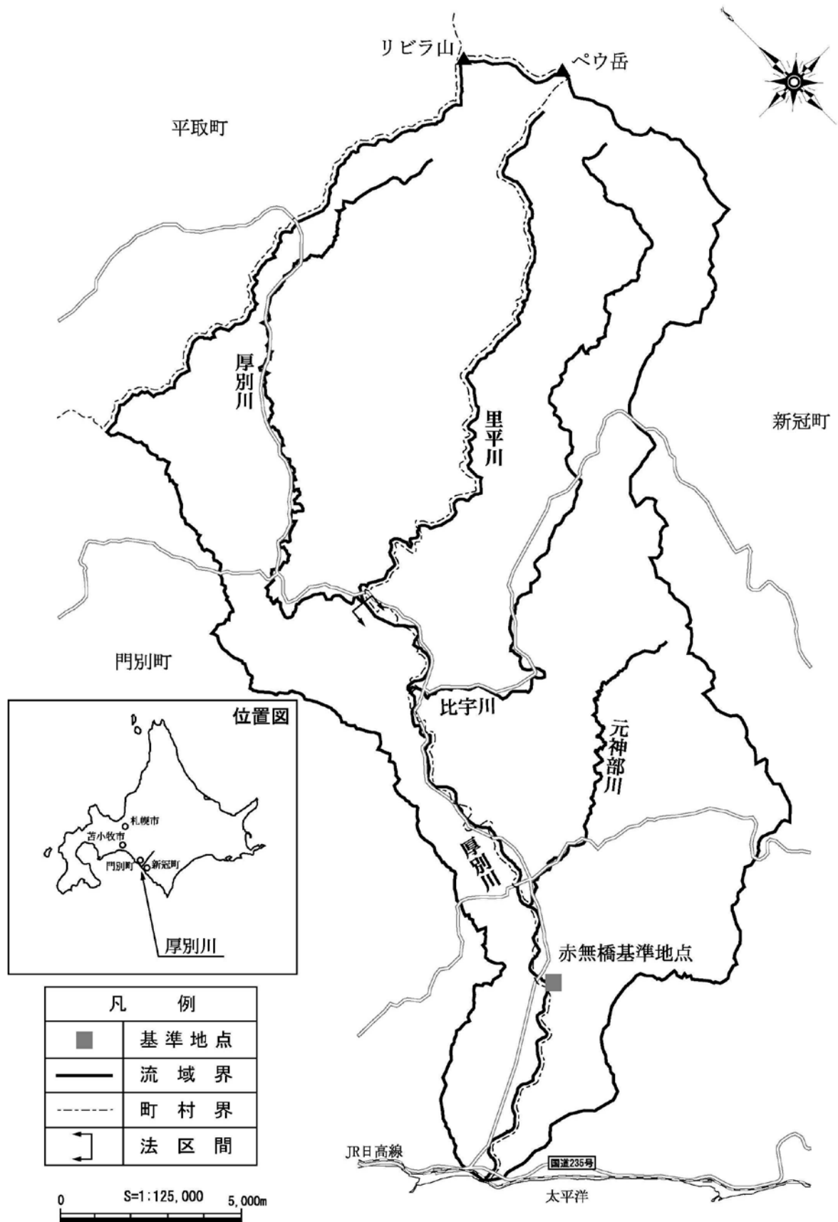
厚別川水系流域概要図
