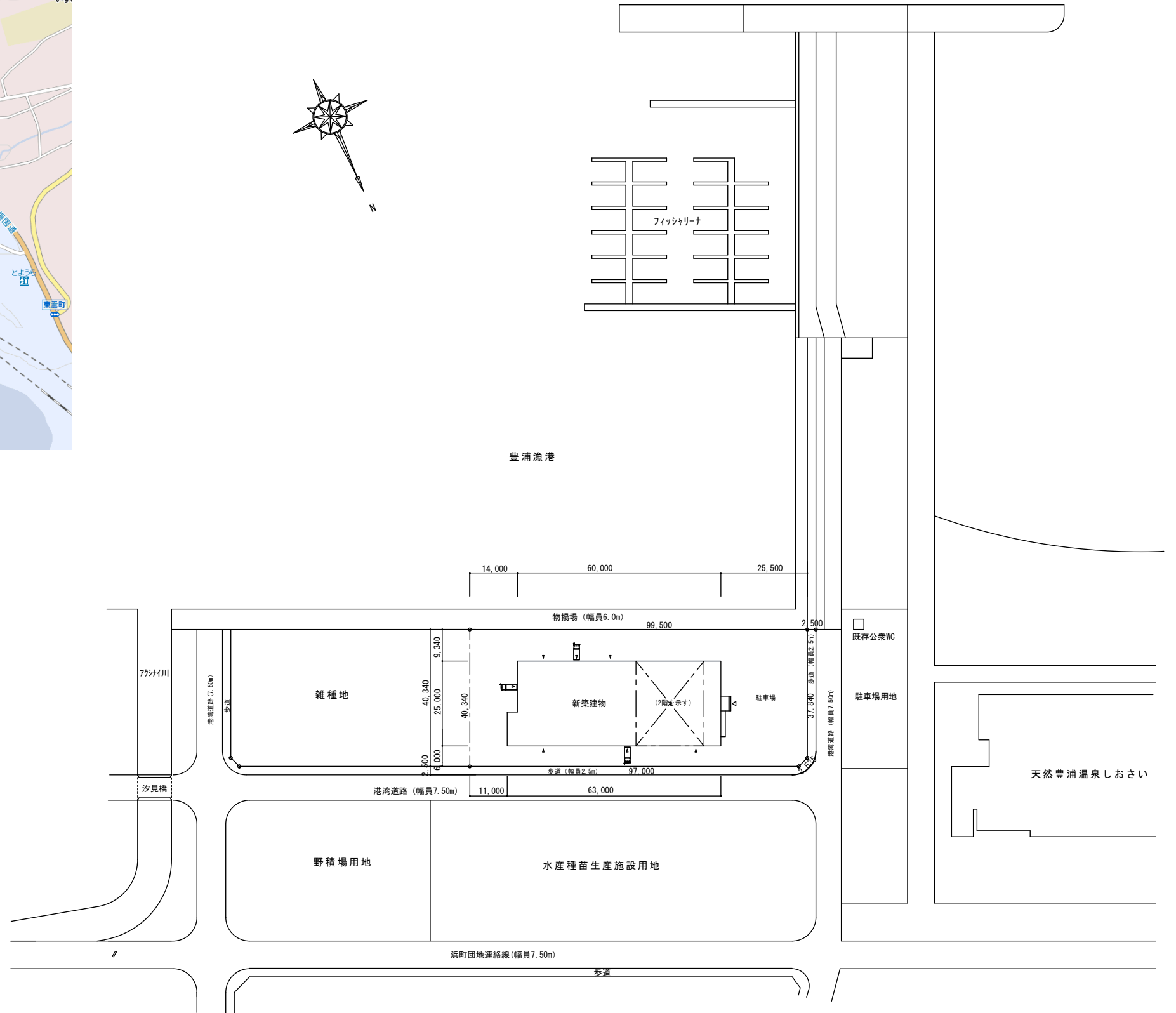
配置図 S=1:1,000
